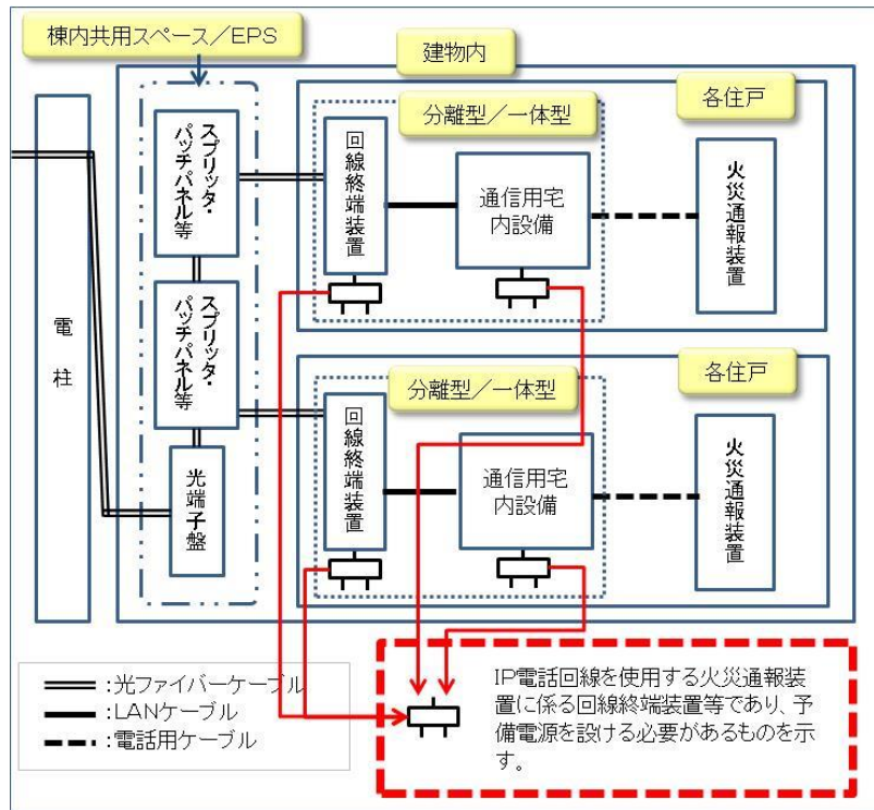
図 1 光配線方式
