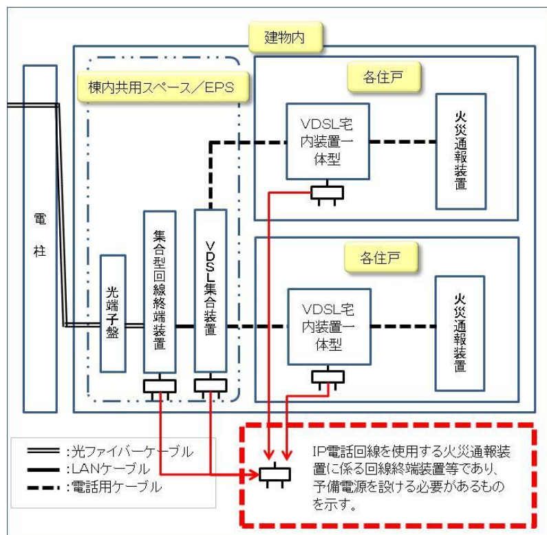
図 2 VDSL 方式
